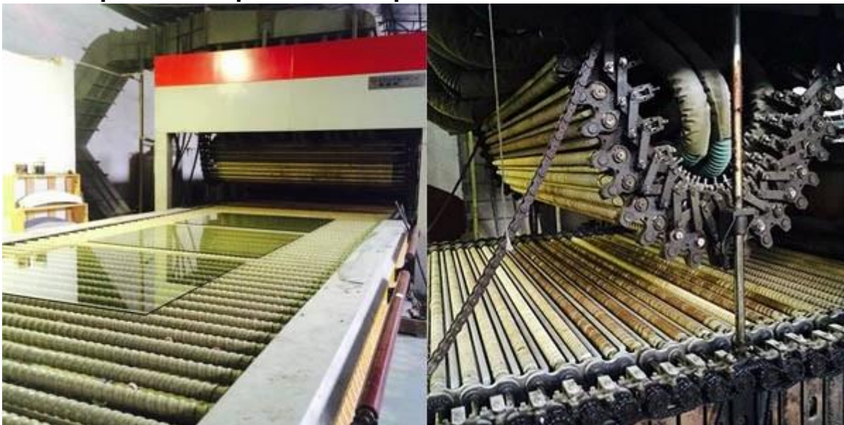
Linea di produzione per vetro temperato 10mm:
